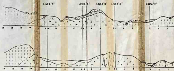
PERFIL LINEA "F"
