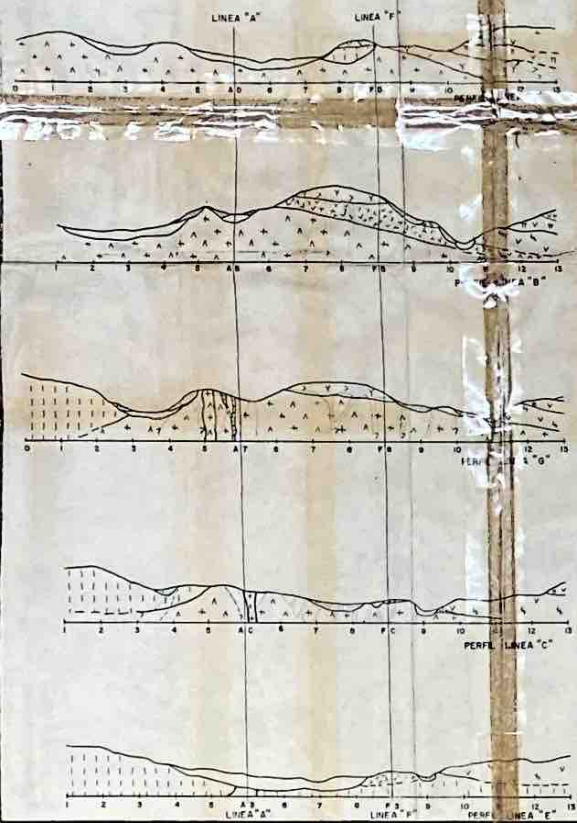
PERFILES GEOLOGICOS ESQUEMATICOS SEGUN LINEAS DE P-1
