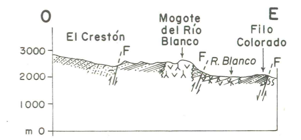
Perfil C-C
