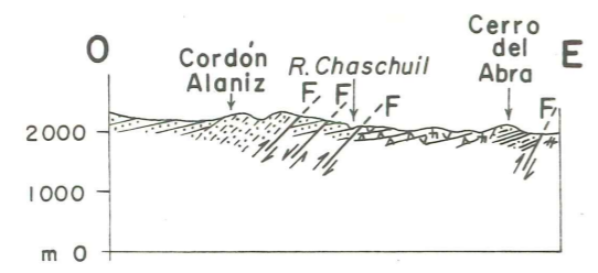
Perfil B-B
