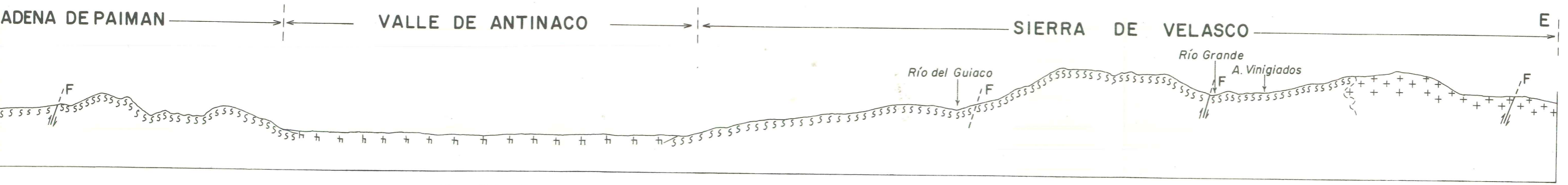
Perfil D-D
