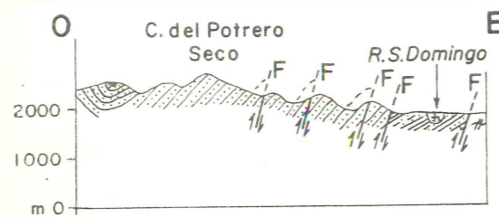
Perfil A-A
